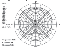
Diagrama polar
