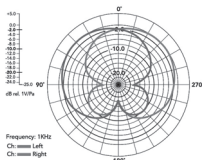
Diagramme polaire
